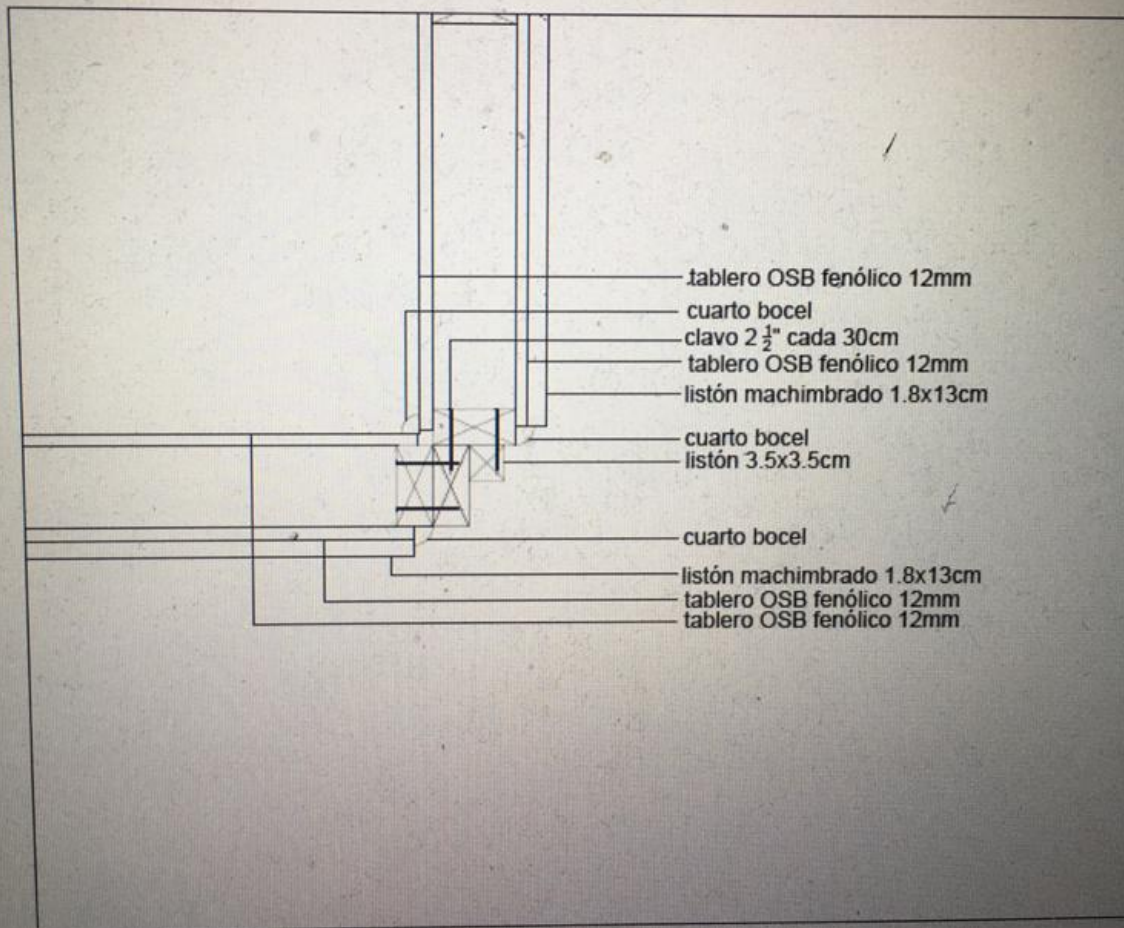
D-6A detalle esquina Esc 1:10
