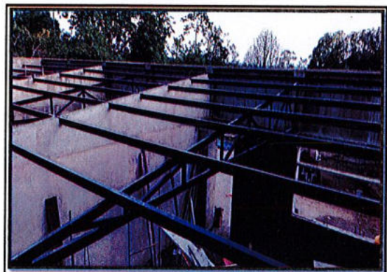
Estructura metálica
