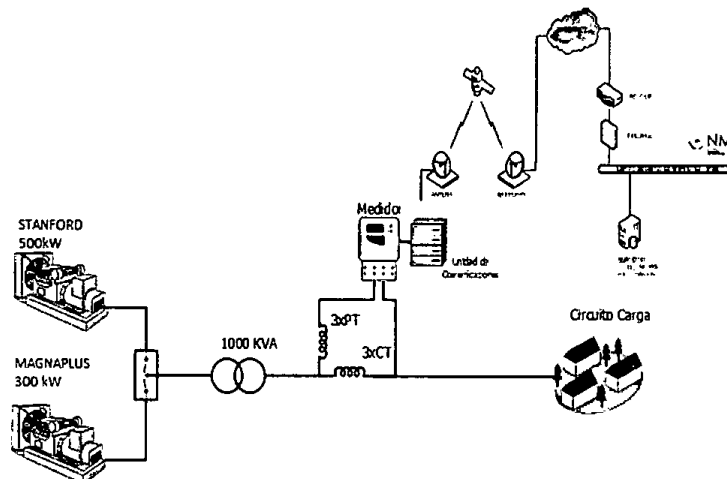
Figura No 1 Esquema del sistema de telemetría y medida en MT
