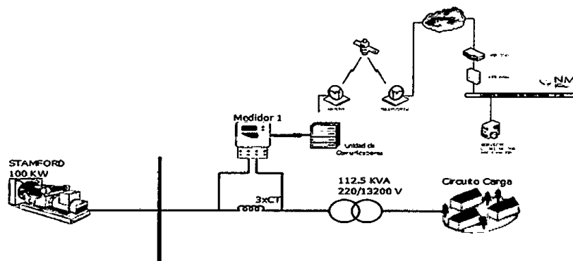
Figura No 2 Esquema del sistema de telemetría y medida en BT
