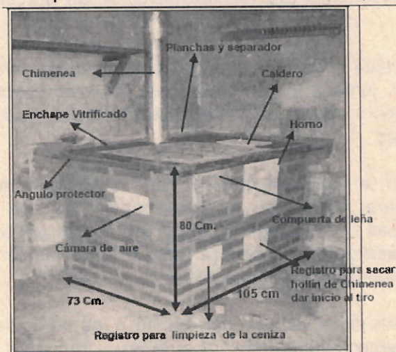
Figura 1. Esquema de la estufa ecoeficiente implementada
