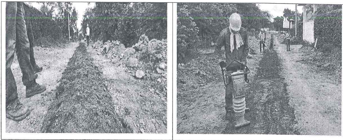
Conexión con pozo 23: (Compactación y extendida de recebo)
