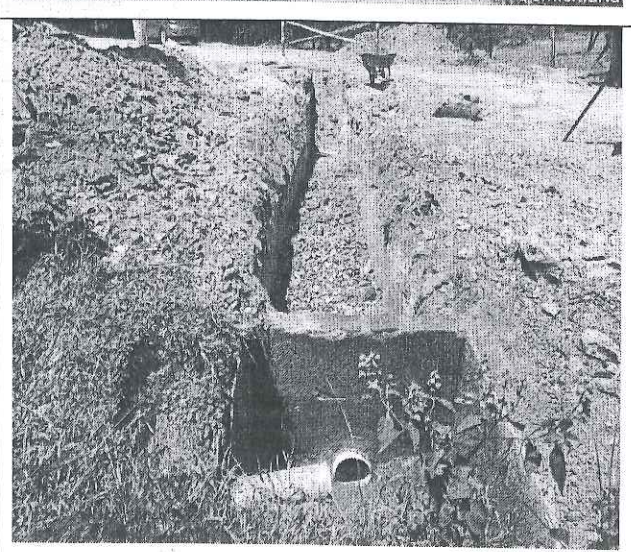
Conexiones domiciliarias- ( Excavaciones, retiro de materiales, instalación de tubería y YEE)
