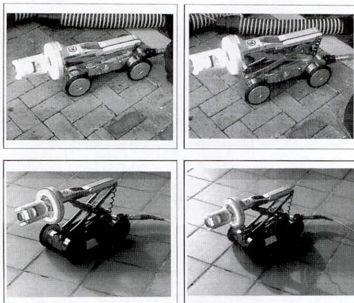
Fotografía 3 Equipo de Inspección de CCTV utilizado en el proyecto (4)
