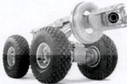
IBAK ORPHEUS en KRA75 con ZSW y ruedas neumáticas
