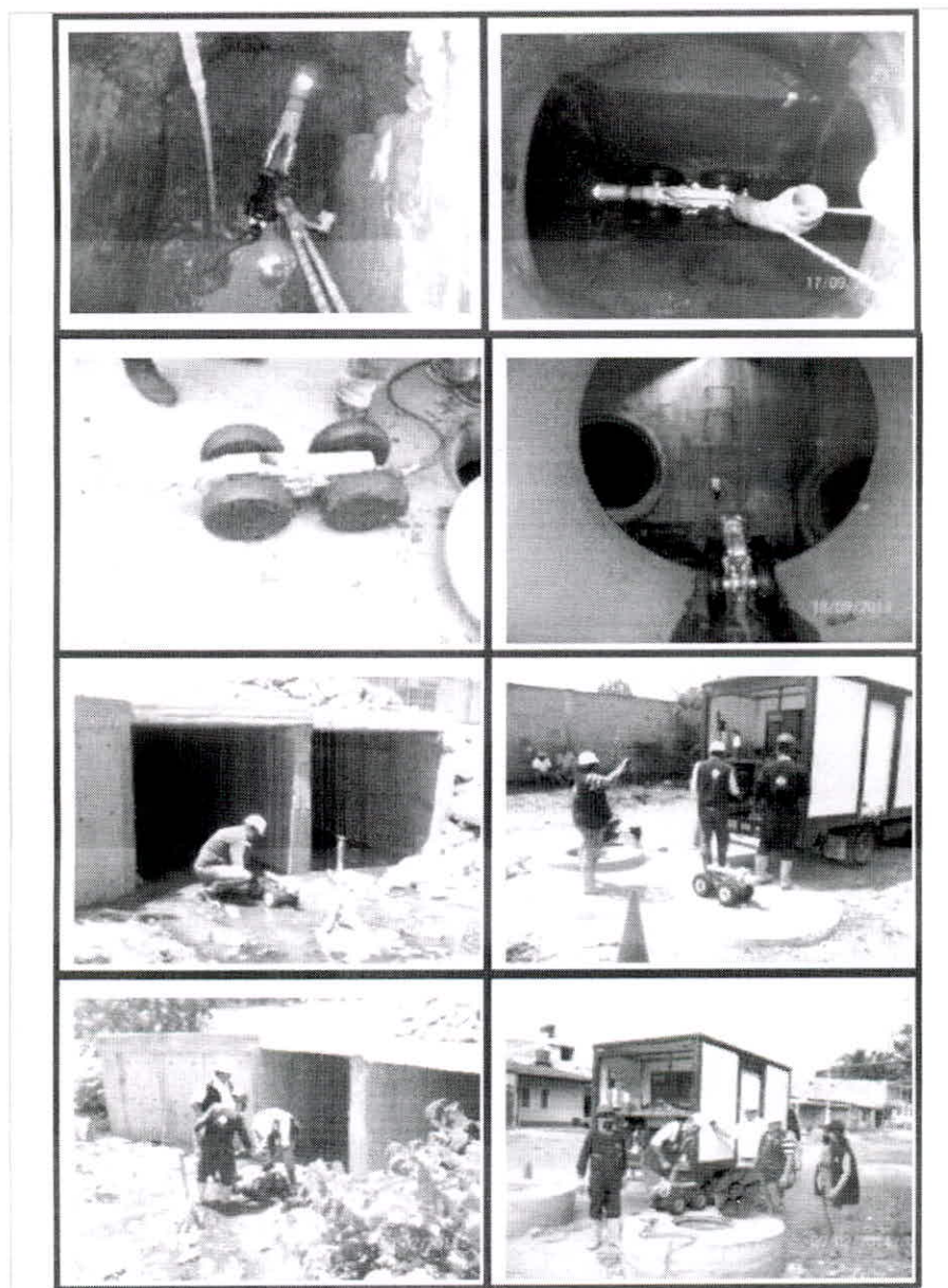
Fotografía 2 Equipo de Inspección de CCTV utilizado en el proyecto (3)
