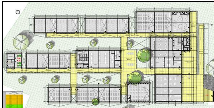
Ilustración 1. Planta general del proyecto – tomado de diseño arquitectónico
