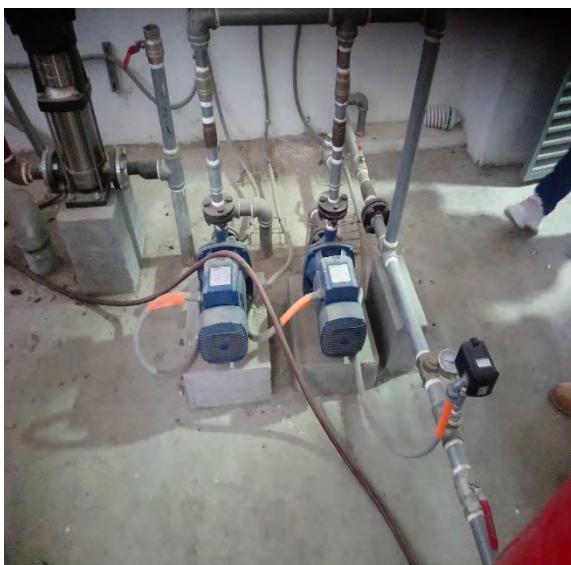
Área de tanque subterráneo y Bombeo.
