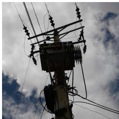
Fotografía 6. Mantenimiento Transformador agroindustrial
