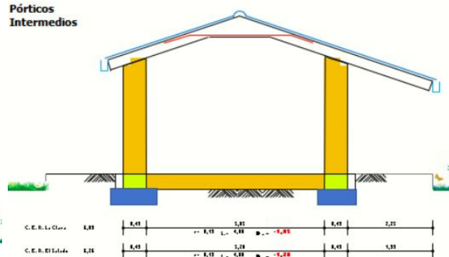
Figura 1. Tipos de pórticos Transversales
