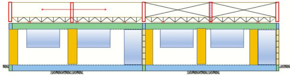
Figura 2. Conformación pórticos longitudinales
