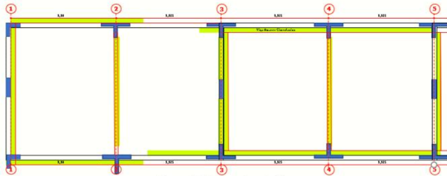
Figura 3. Diafragma cimentación
