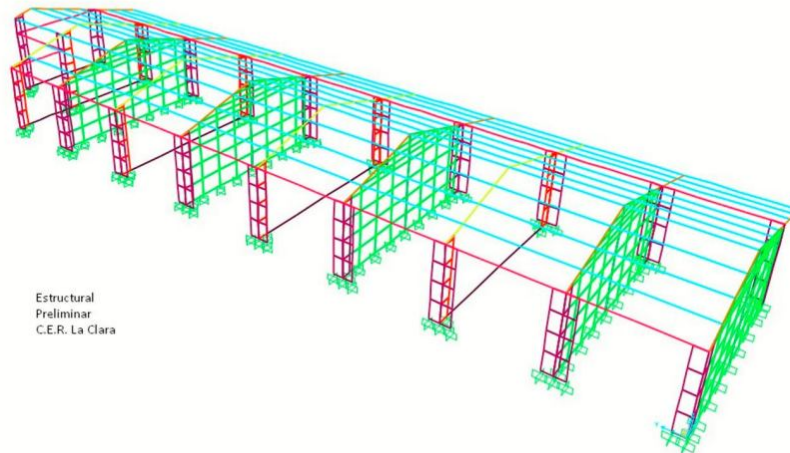
Figura 4: Modelamiento en SAP2000 de la estructura del C. E. R. La Clara
