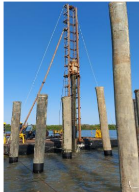
Pilotes hincados en el frente tierra (Modulo 2) semana 3.
