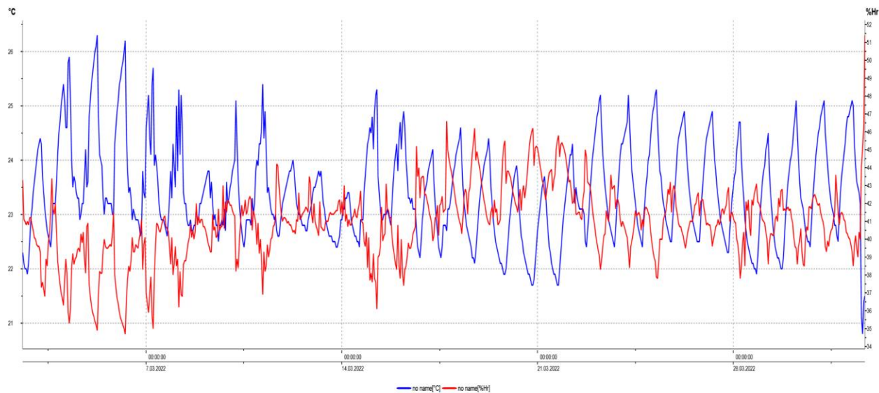
Grafica 3. Variaciones variables Hr% y T° mes de marzo.
