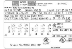
Fig. No. 3. Placa característica de motor 1
