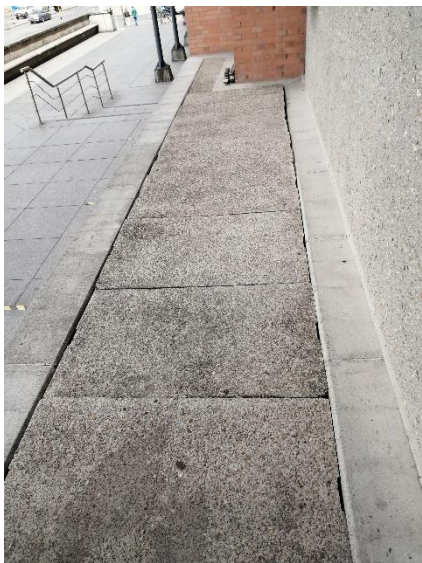
Fotografía N° 9: Losas en concreto dilatadas
