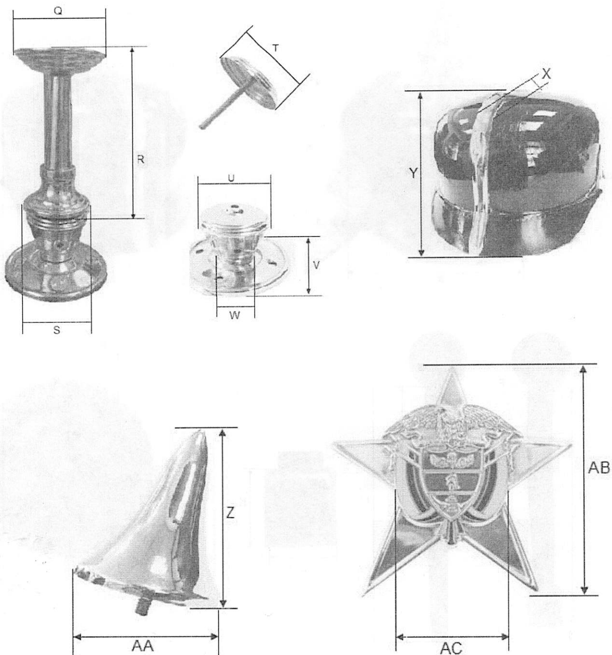
Figura ilustrativa No. 3 Cotas Casco de Ceremonia
