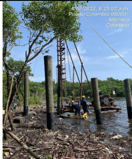
Hincado de módulo 13
