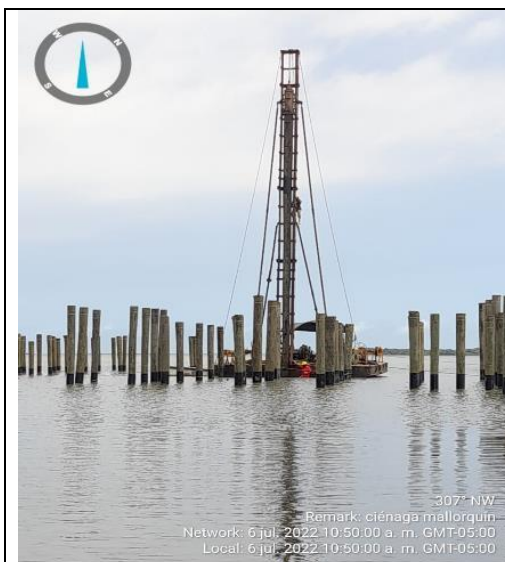
Hincado de módulo 46.
