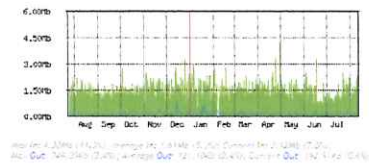
Imagen 10. Graficas de monitoreo y consumo – Planta de beneficio animal – (PBA)
