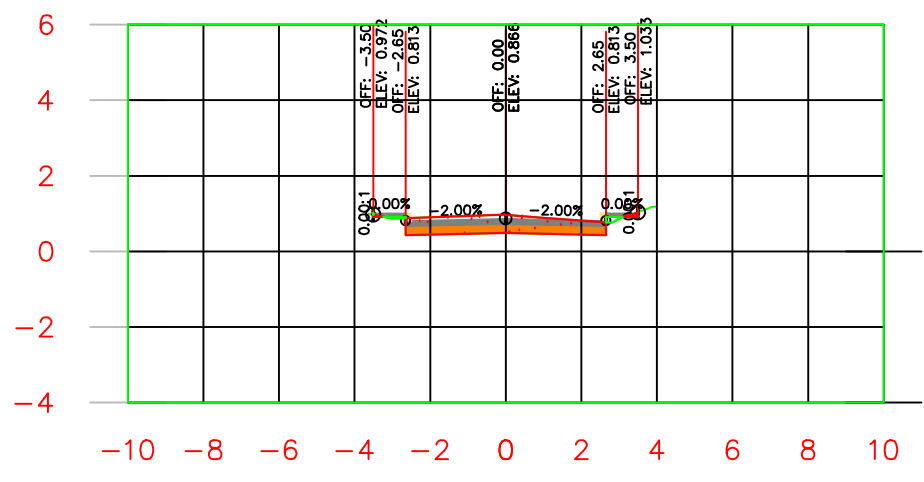
K0+095.00
