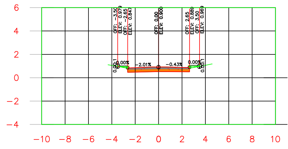
K0+025.00
