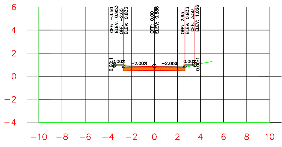
K0+055.00
