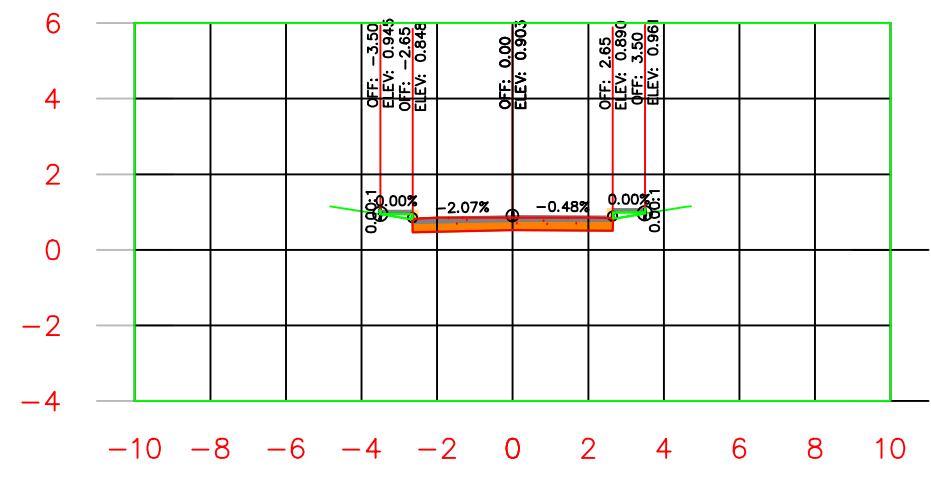
K0+020.00
