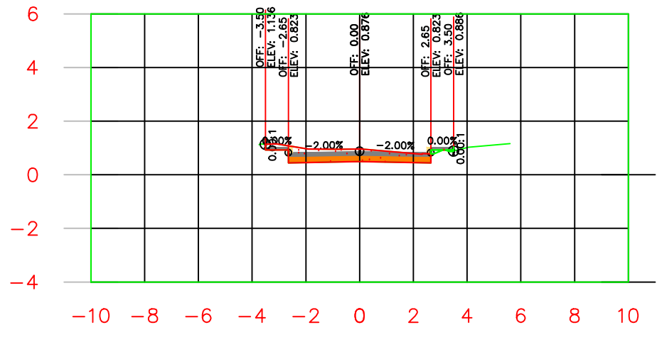
K0+075.00
