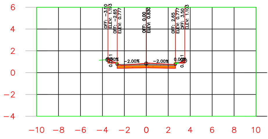
K0+170.00
