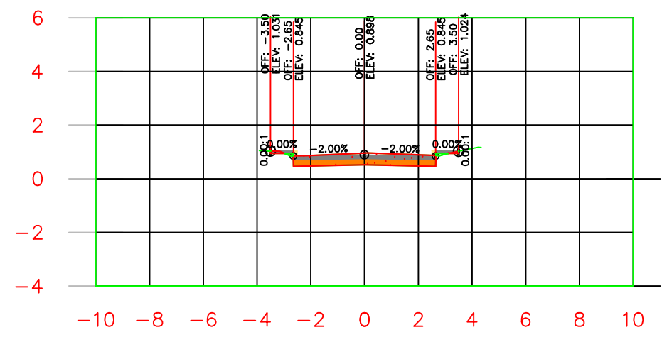
K0+030.00
