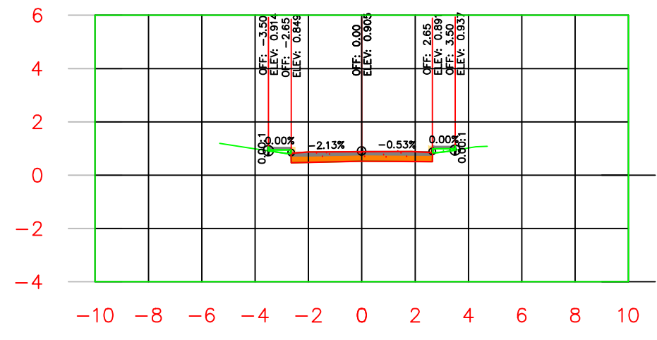
K0+015.00
