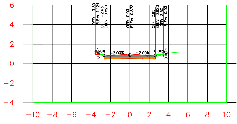
K0+080.00
