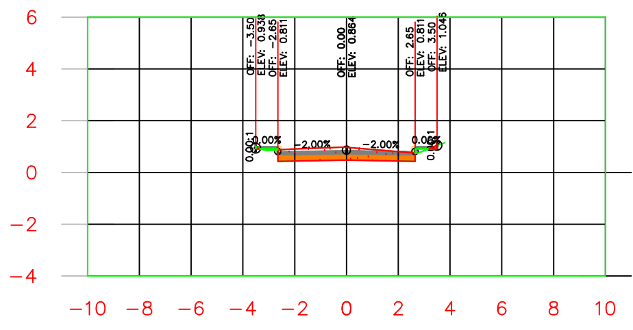
K0+100.00
