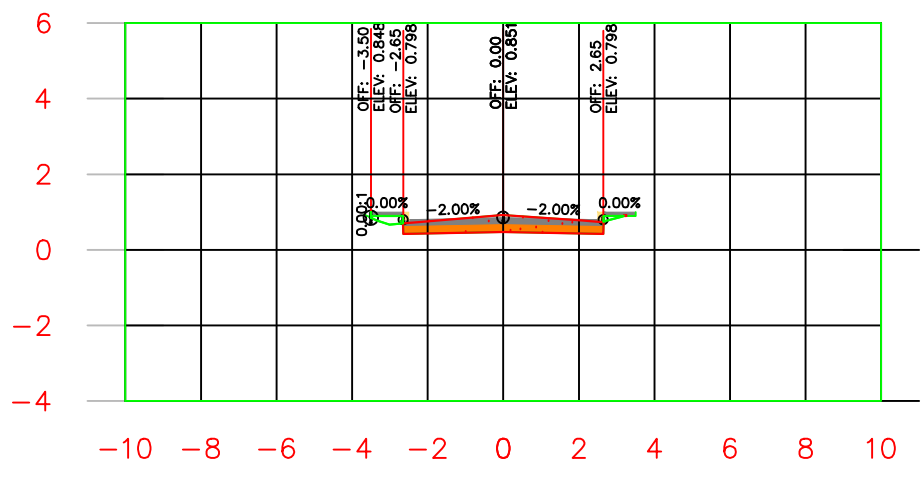
K0+125.00
