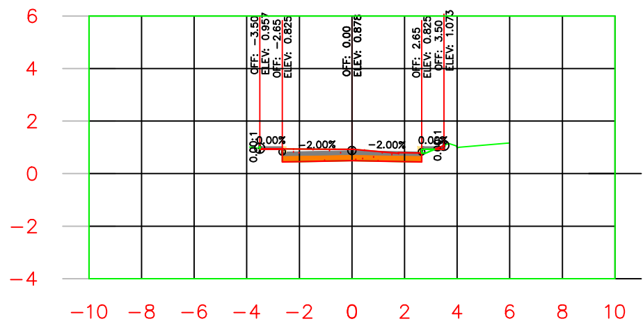
K0+070.00
