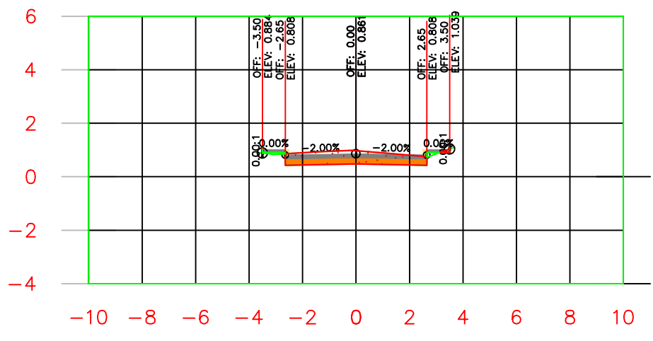
K0+105.00
