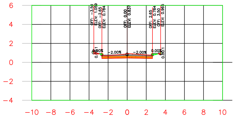
K0+155.00
