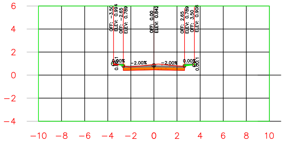
K0+145.00
