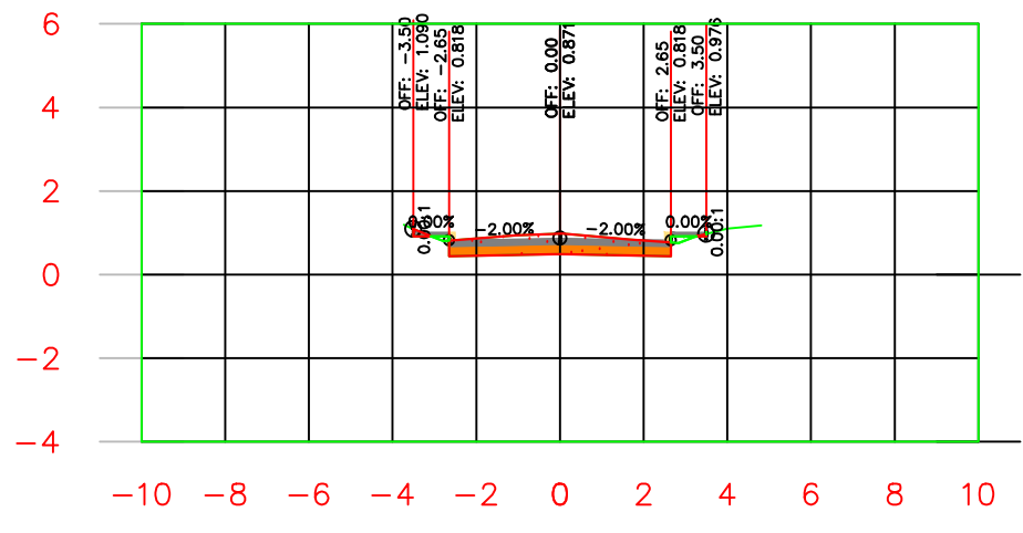
K0+085.00
