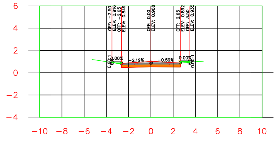
K0+010.00
