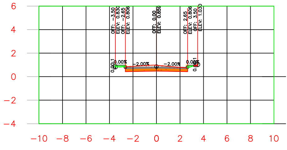
K0+110.00
