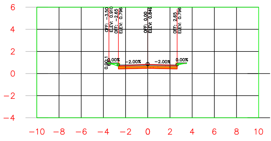
K0+130.00
