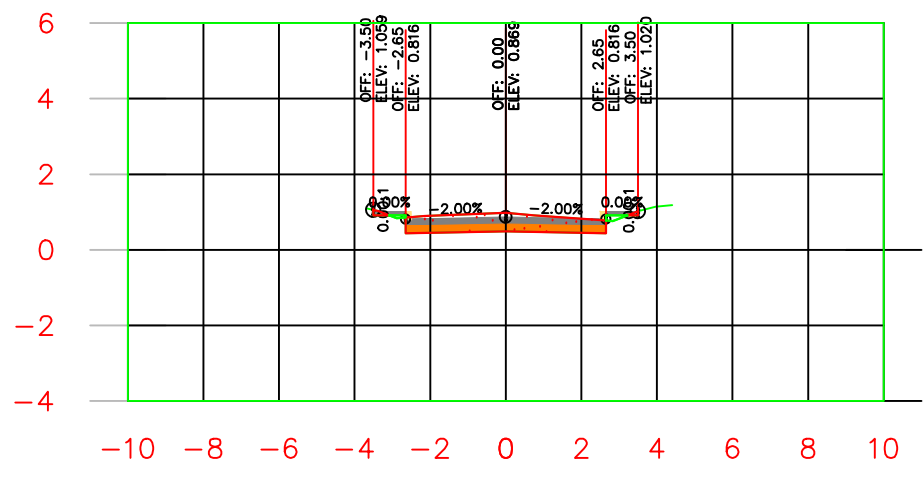
K0+090.00
