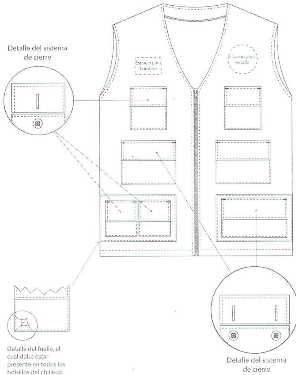
Figura 1. Vista frontal chaleco habano para Unidades Tácticas y detalles vista superior del bolsillo inferior izquierdo y derecho.
