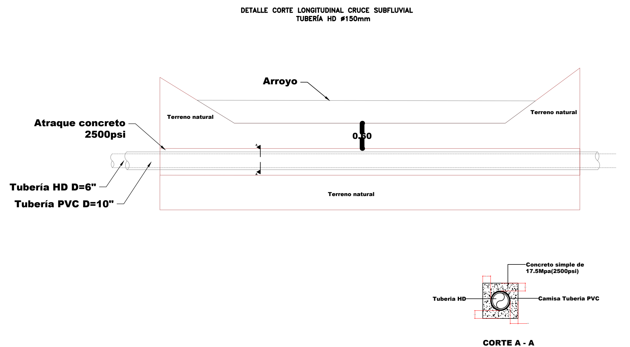
CORTE A - A
