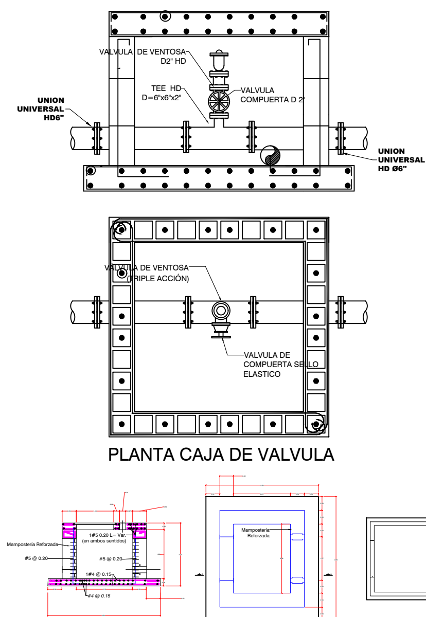
CAJA VENTOSA SOBRE LA LINEA DE CONDUCCION
