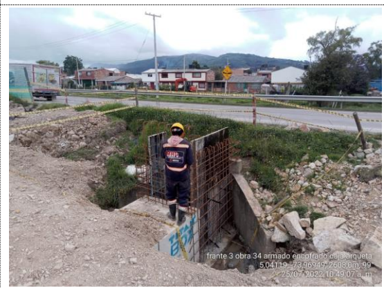
Obra No 34 Box culvert 1x1 K4+686 armado de acero y encofrado caja arqueta (25/07/22)
