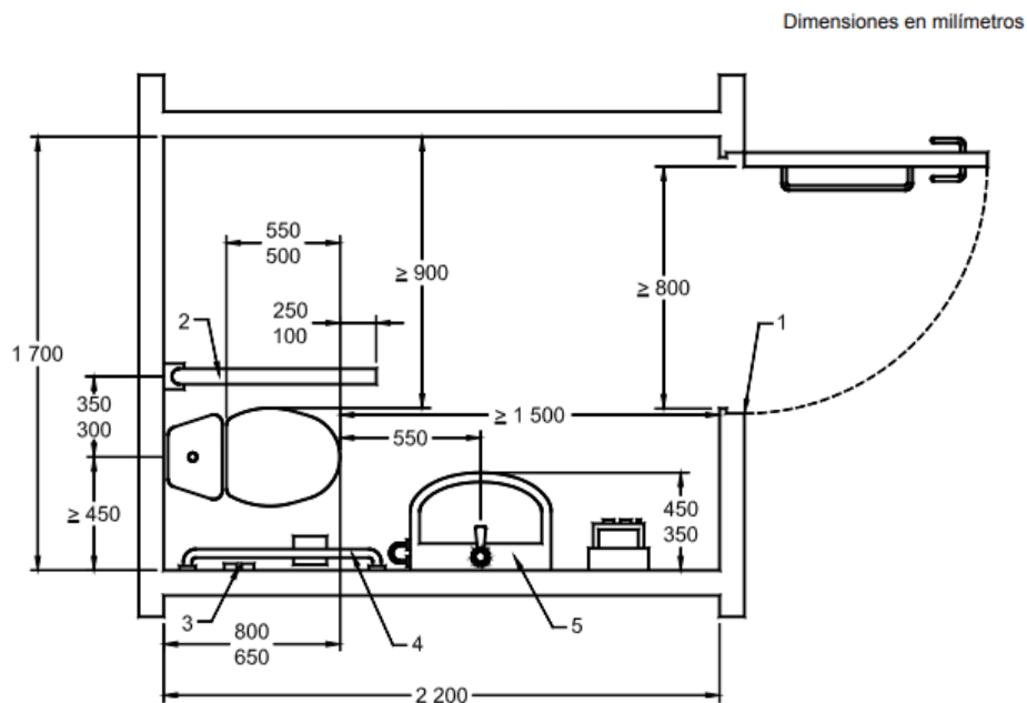
Imagen 3. Opción C (con una barra de agarre horizontal y abatible, y otra barra de agarre horizontal en la pared)
