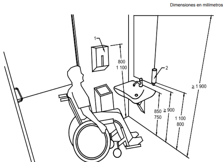
Imagen 4. Ubicación de lavamanos para baño de ciudadanos en silla de ruedas
