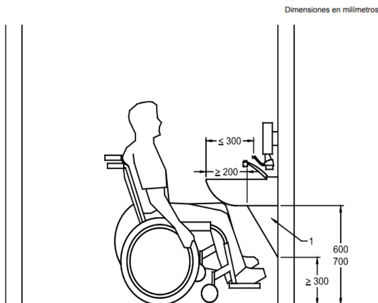
Imagen 5. Altura de lavamanos para baño de ciudadanos en silla de ruedas
