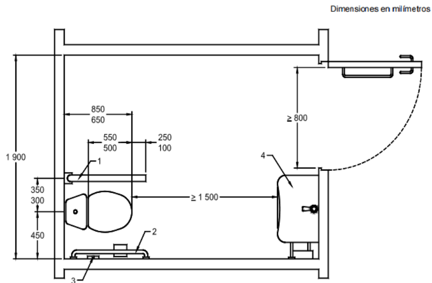
Imagen 2. Opción B (con una barra de agarre horizontal y abatible, y otra barra de agarre horizontal en la pared)
