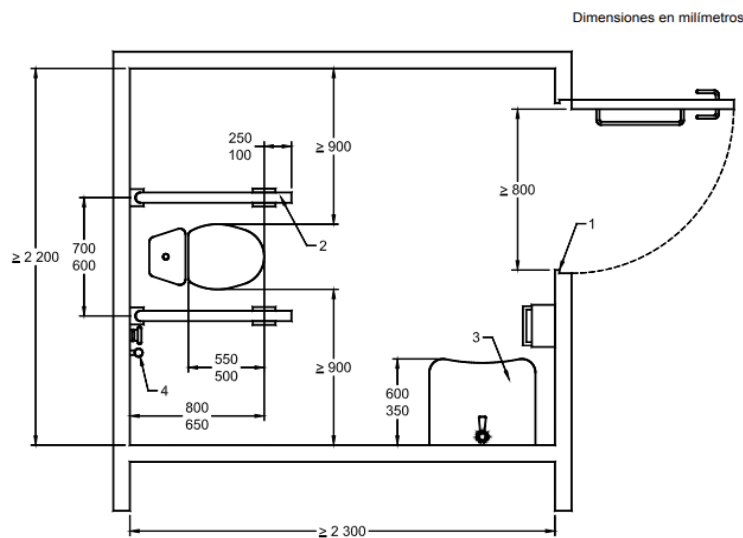
Imagen 1. Opción A (barras de agarre horizontal y abatible a ambos lados del inodoro)
