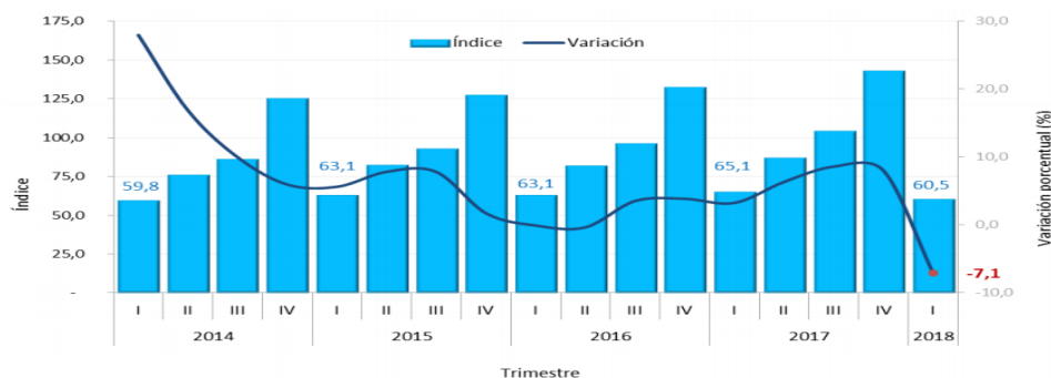
Gráfico 2. Pagos en obras civiles (índice/ variación anual) Total nacional 2014 - 2018 pr (I trimestre) – serie empalmada
