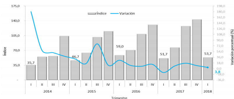
Gráfico 13. Indicador de obligaciones en otras obras de ingeniería (índice / variación) Total nacional 2014 - 2018 IV (I trimestre) – serie empalmada
