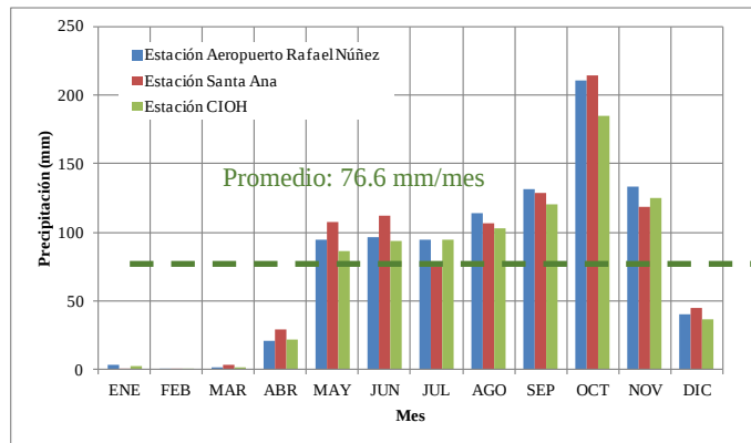
Figura 5.- Valores Totales Mensuales de Precipitación de estaciones con registros de lluvias circundantes al Distrito de Cartagena.
