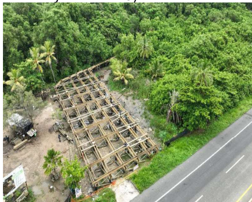
Instalación de vigas laminadas Estación III.
