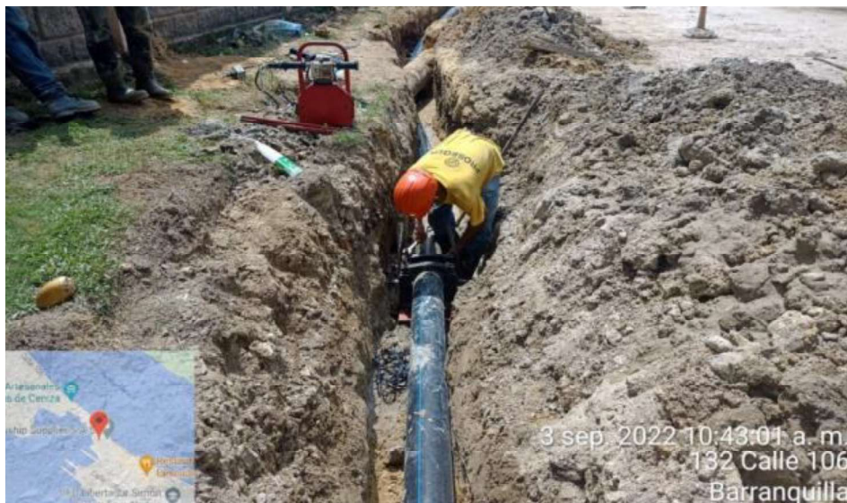
Imagen 35: Excavación e instalación tubería PEAD.
