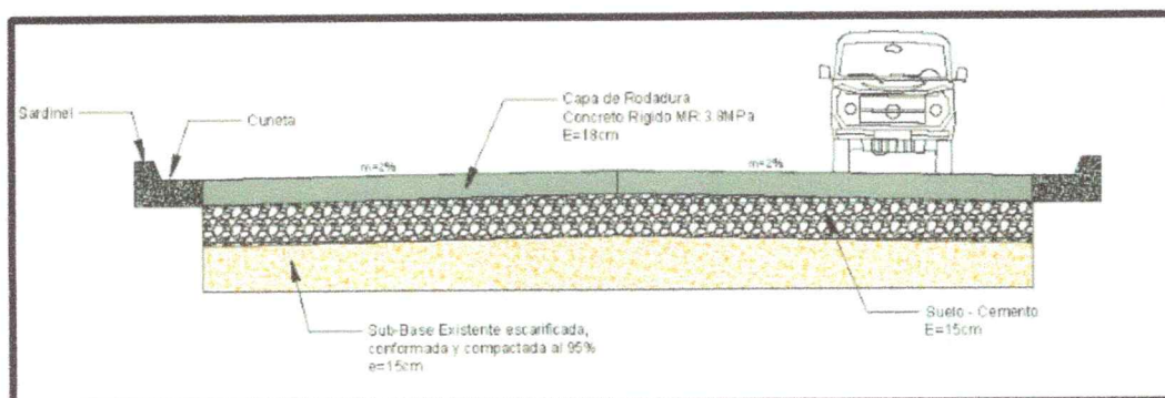
Imagen 14. Perfil de la sección transversal del pavimento en concreto Estructura Existente – Alternativa 2
