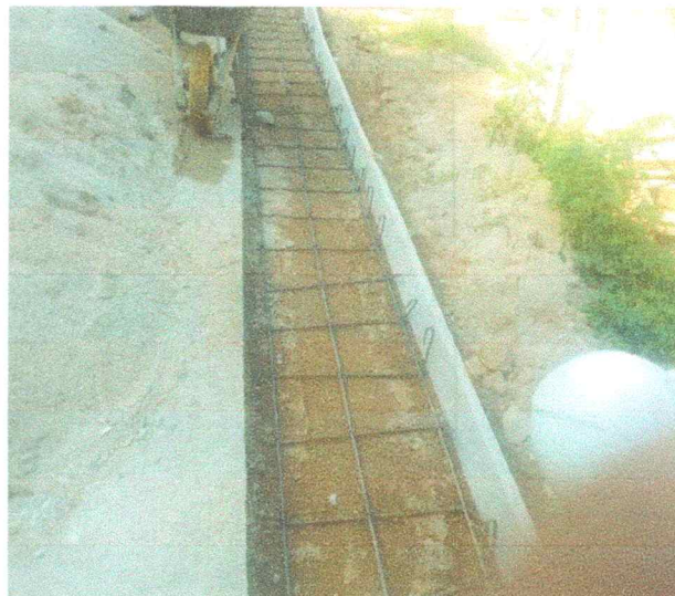
FIGURACION DE ACERO PARA CUNETAS
