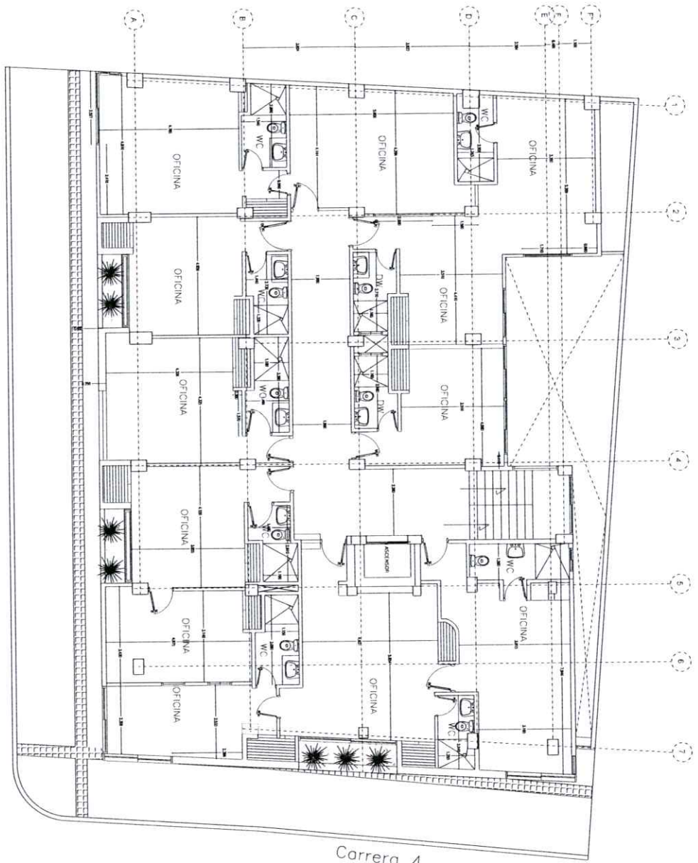
Colle 27 PLANTA ARQUITECTÓNICA 5TO. PISO
