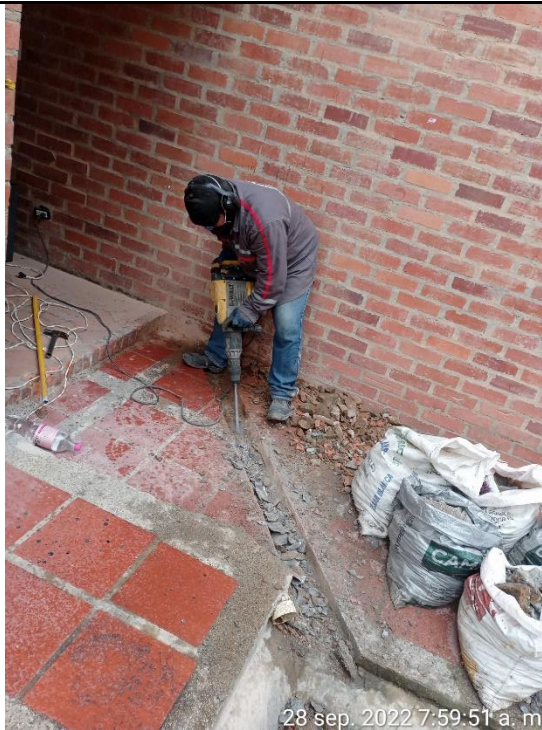
Desmante enchape para instalación de bajantes aguas lluvias en PVC.
