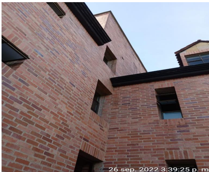
Estado final alfajia en el bloque alojamientos C
