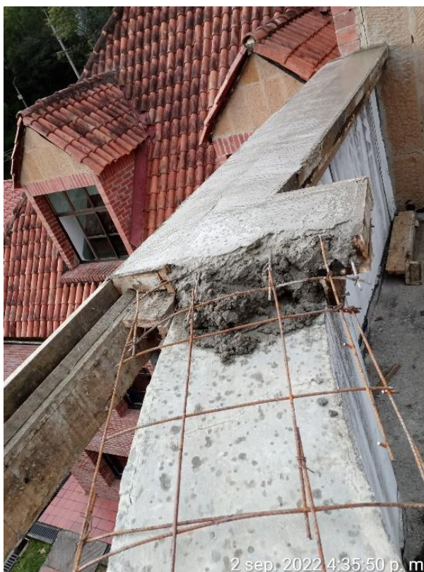
Formaleta e Instalación de alfaja en punto fijo bloque academino N°1
