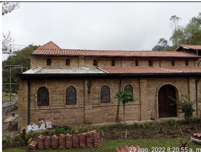
Desmante teja de barro ala derecha de la capilla, así mismo de listones en madera podridos.
