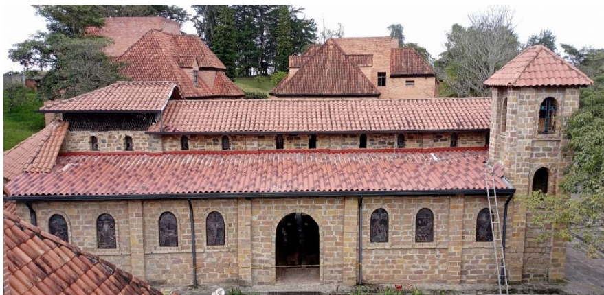
Aplicación de mortero impermeabilizante con bronco repelente y tela de refuerzo impermeabilizante.
