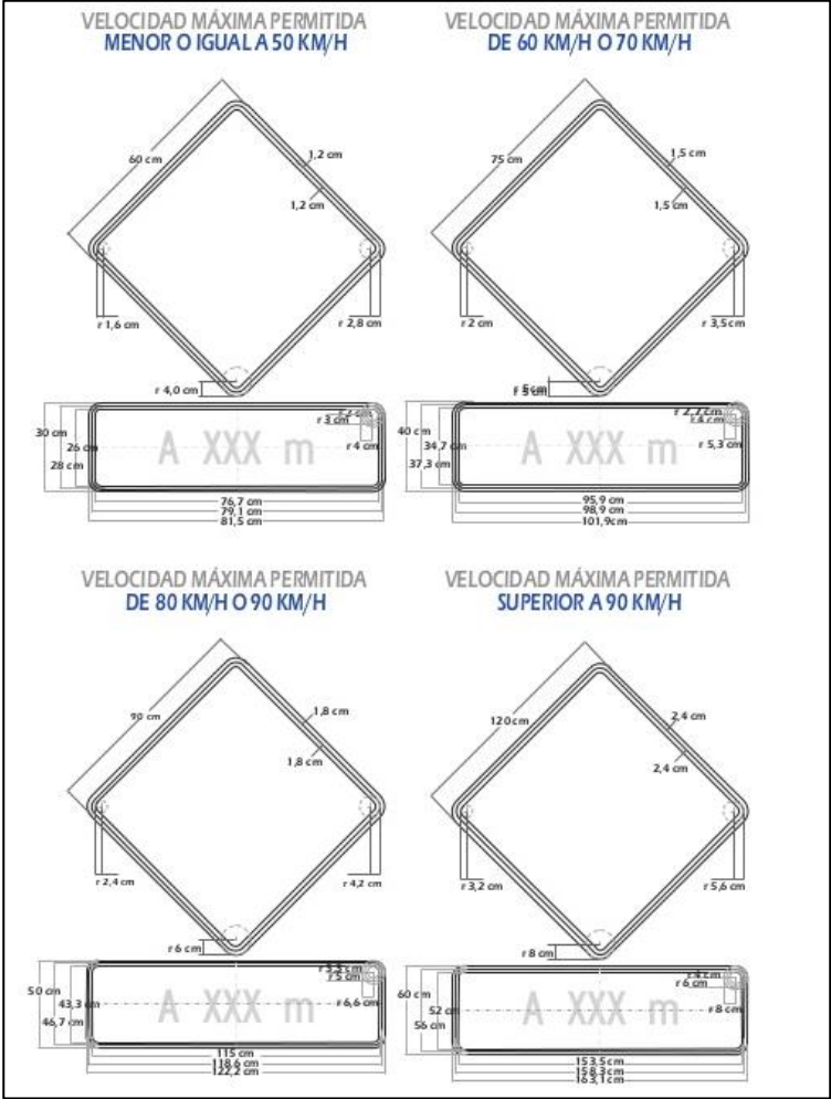
Ilustración 3: Dimensiones señales preventivas para obras
