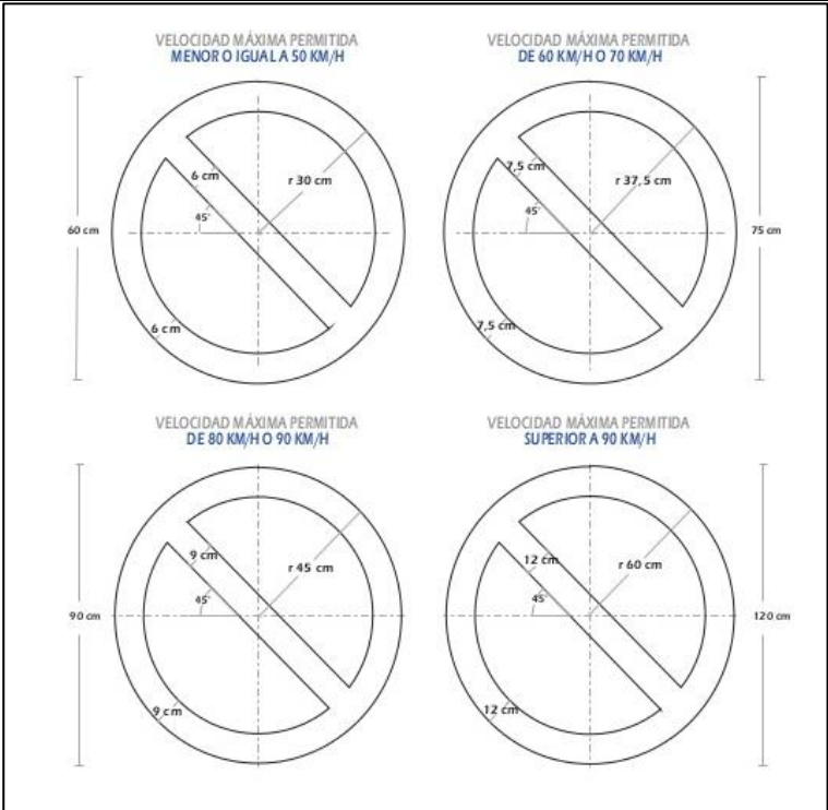
Ilustración 2: Dimensiones señales reglamentarias en obra
