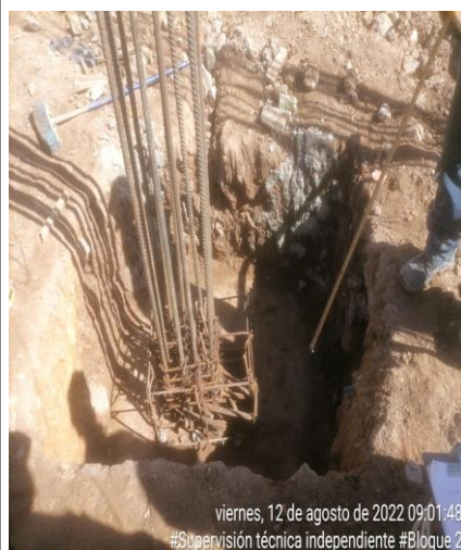
Página 9 de 22 Bloque 2: Refuerzo para dados eje H-I entre 18-19
