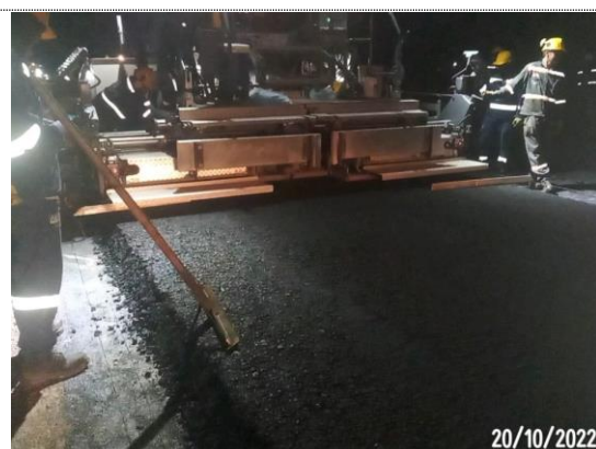
K2+200 – K2+350 instalación y compactación de BTA carril derecho (20/10/22)
