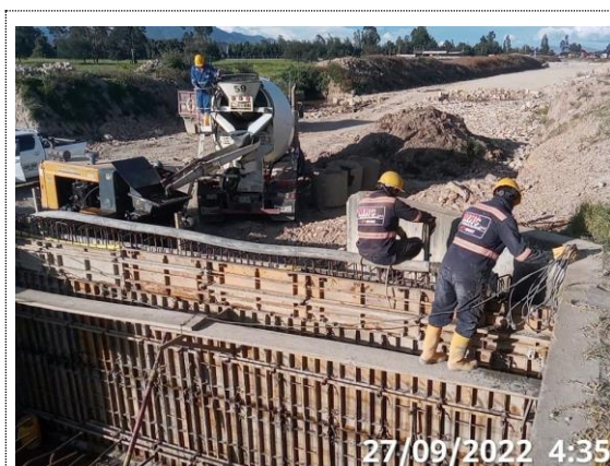
Obra No. 6 Pasaganado 3X3 K1+069 fundida vástago norte módulo 3 (27/09/22)
