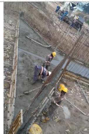
Obra No. 6 Pasaganado 3X3 K1+069 fundida de placa inferior de encofrado (02/09/22)
