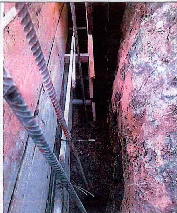
Instalación de hierros para construcción del muro (Agricol)
