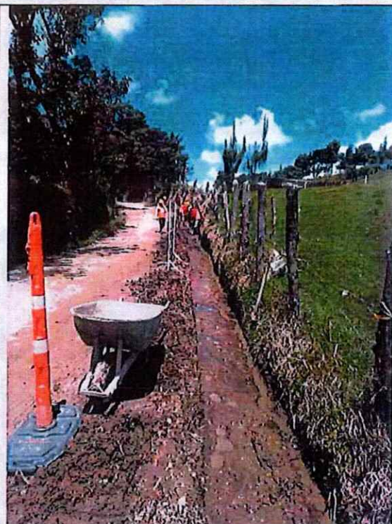
Excavación de cunetas
