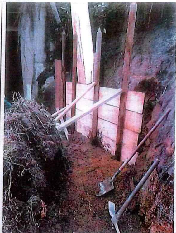
Formaleta de muro de contención (Agricol)
