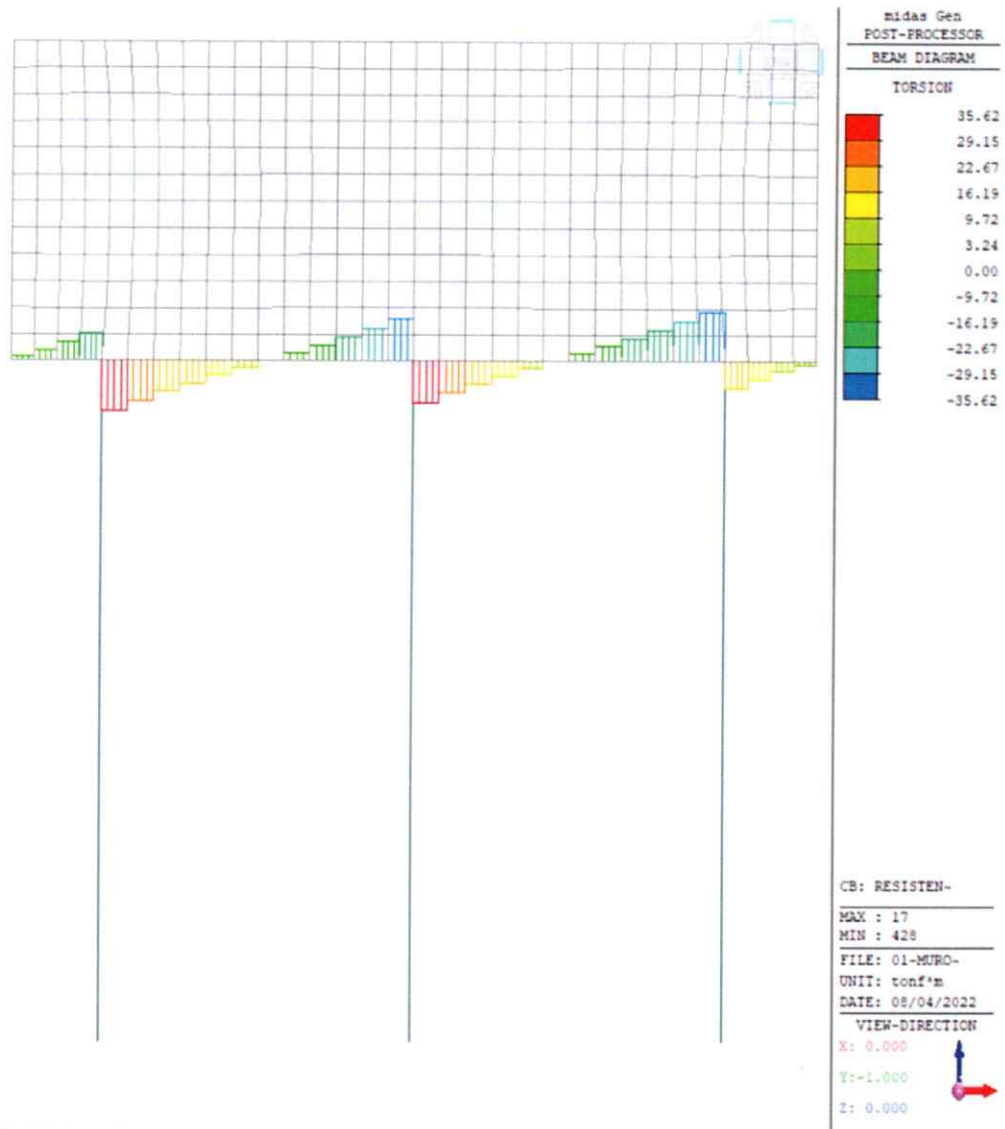
Figura 17. Torsión (envolvente). [ton-m]
