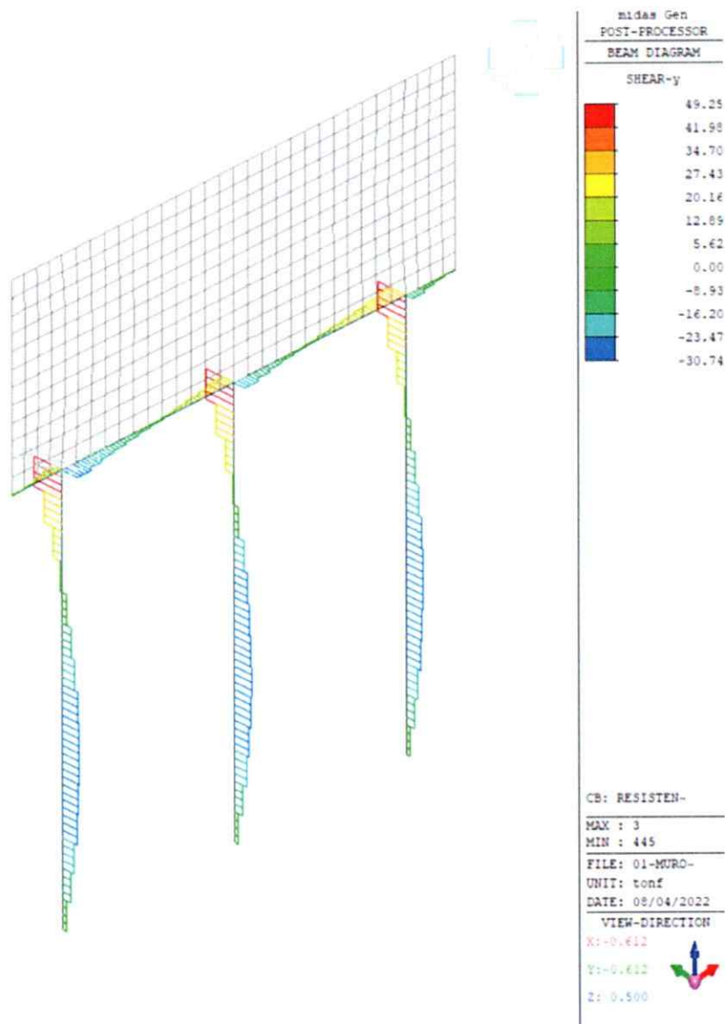
Figura 16. Cortante 3-3 viga y pilas (envolvente). [ton]
