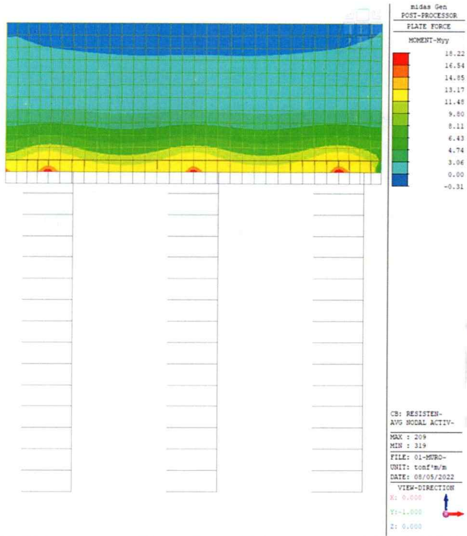
Figura 21. Momento Myy max (envolvente). [ton-m/m]
