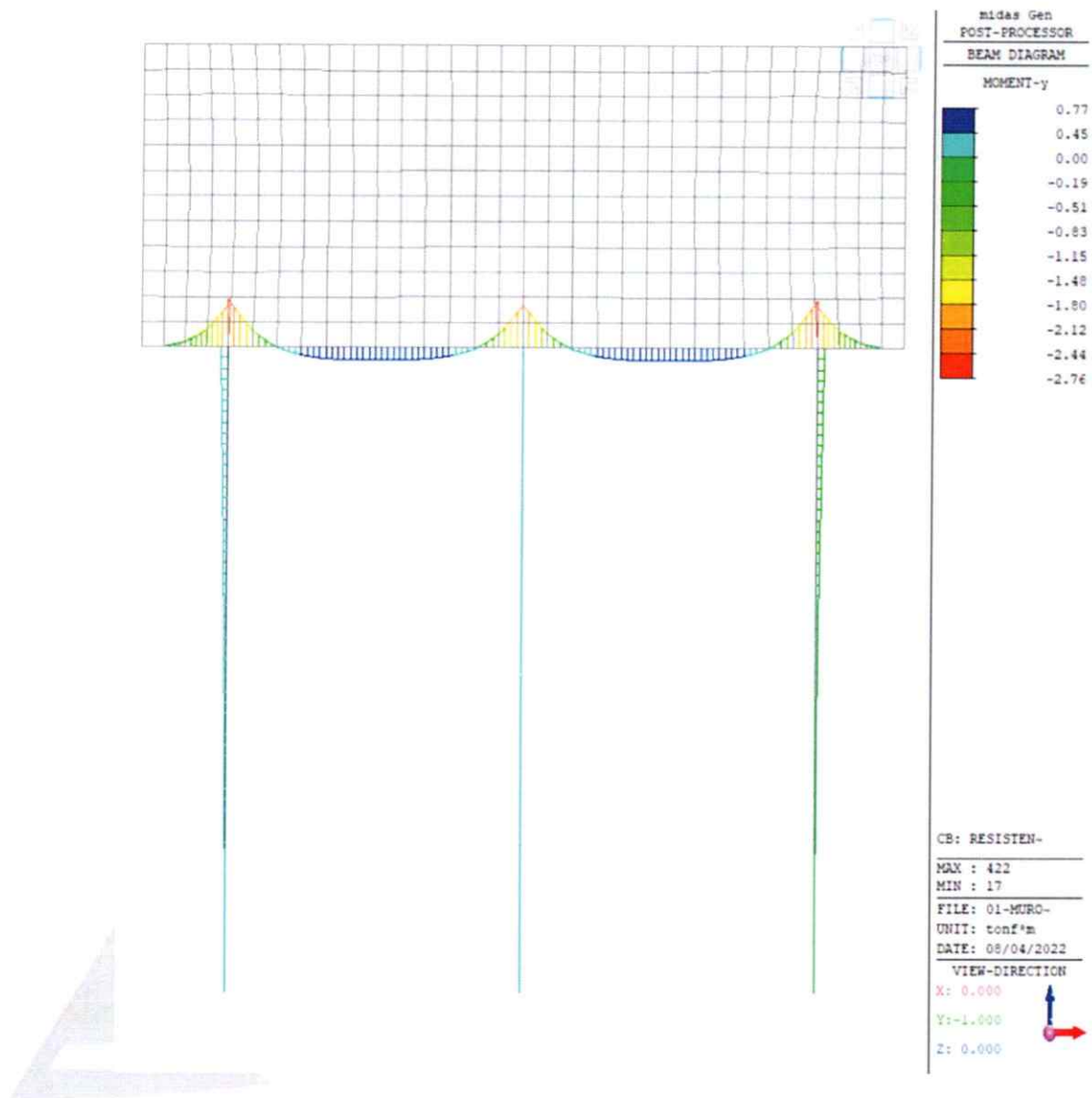
Figura 19. Momento 3-3 viga y pilas (envolvente). [ton-m]
