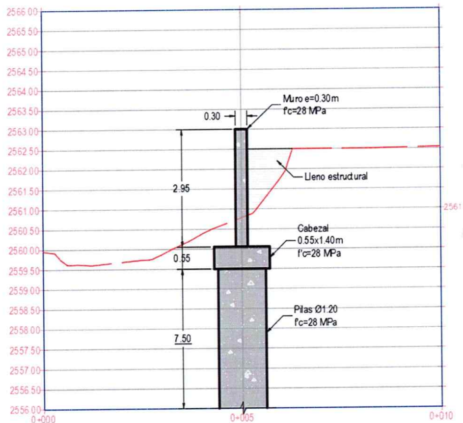
Figura 2. Sección transversal muro de contención
