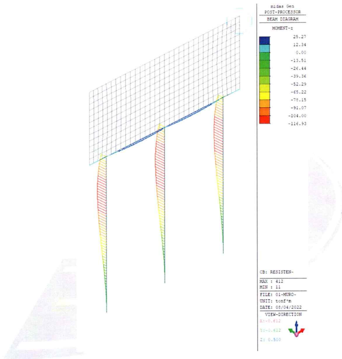
Figura 18. Momento 2-2 viga y pilas (envolvente). [ton-m]
