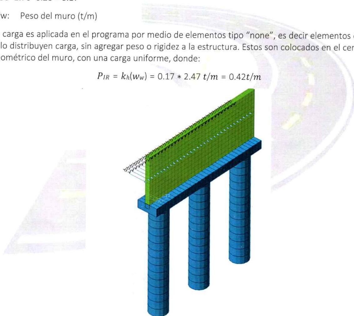
Figura 13. Fuerza inercial PIR [ton/m]
