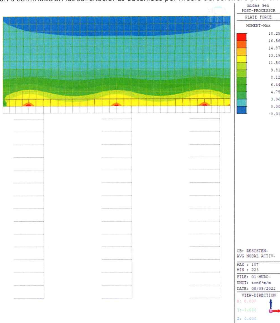
Figura 20. Momento Mxx Max (envolvente). [ton-m/m]
