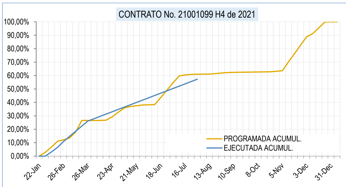
Figura 8.4 Avance programado vs avance ejecutado en semanas
