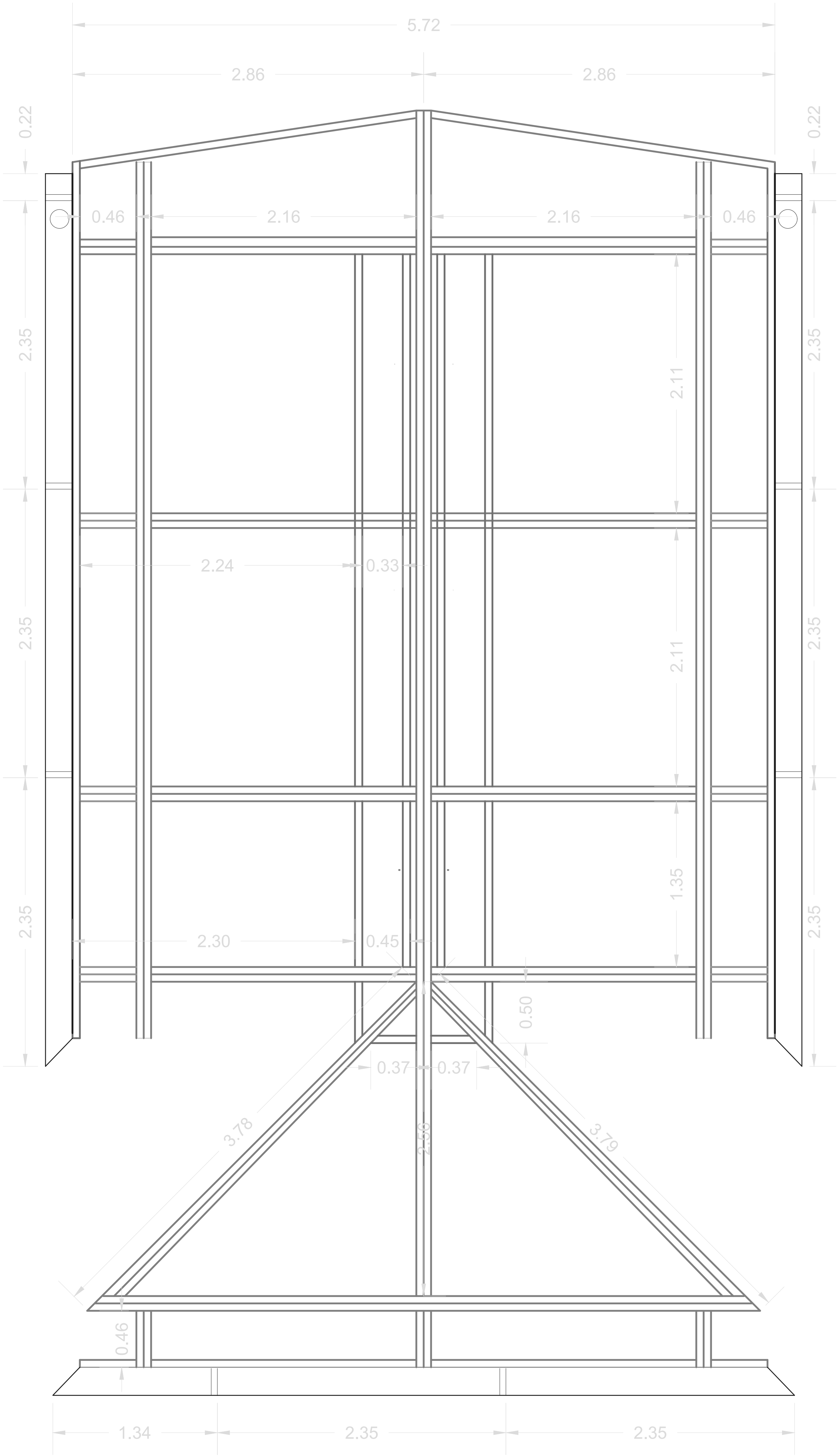
ESTRUCTURA Y CORREAS
