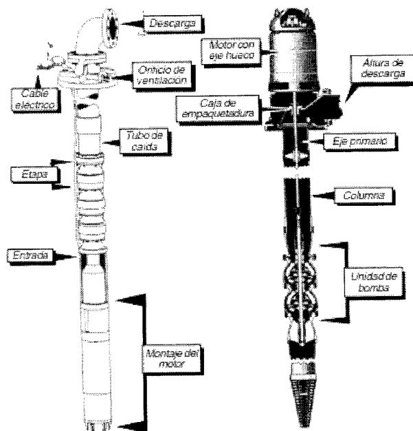
Turbina del eje de transmisión
