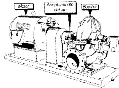
Bomba horizontal de doble aspiración
