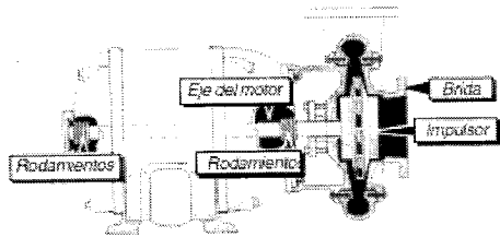
Bomba horizontal - Acoplada en forma compactada
