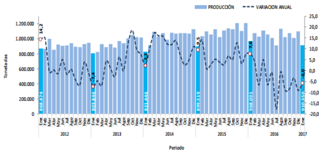
Gráfico 6. Producción de cemento gris Variación anual 2012 (enero) - 2017 (enero) P
