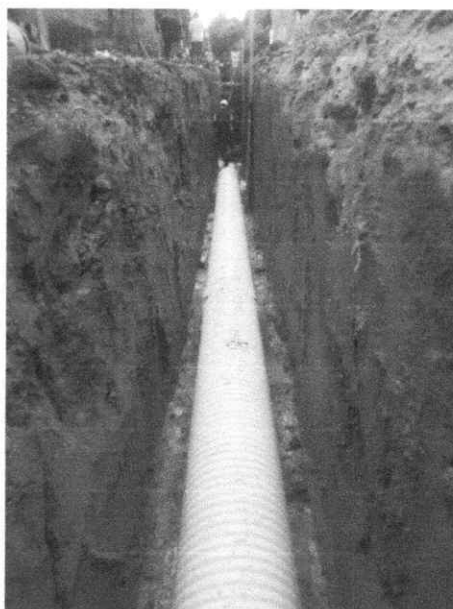
FOTOFAGRIA 8- Instalación tubería Pvc de 16"
