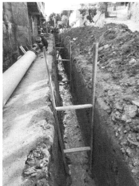
FOTOFAGRIA 6- Entibada
