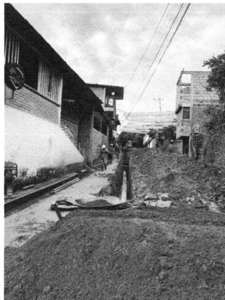
FOTOFAGRIA 10- Instalación tubería Pvc de 16"
