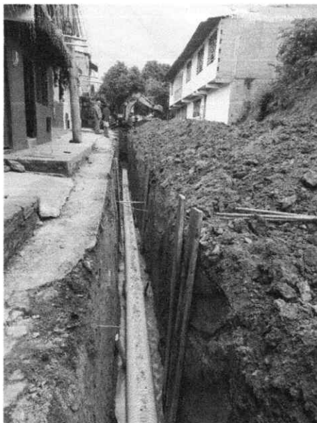
FOTOFAGRIA 9- Instalación tubería Pvc de 16"
