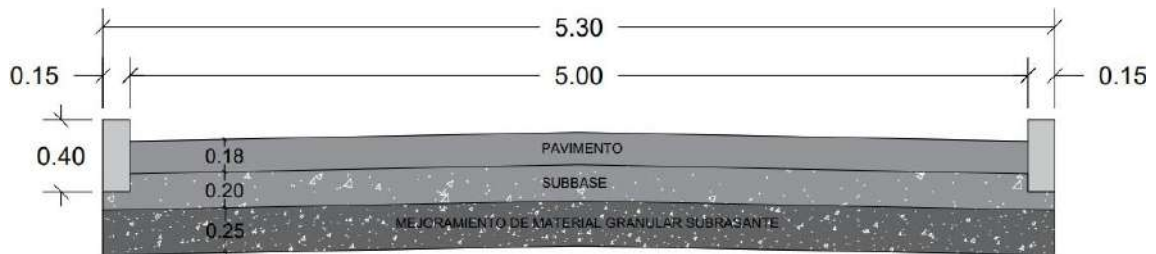
Figura No 2. Sección de vía. Fuente elaboración propia.
