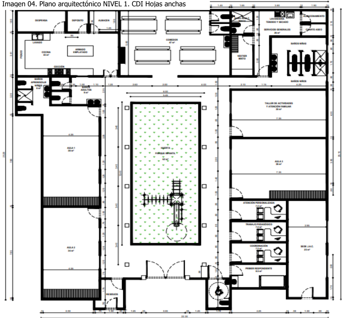
Imagen 04. Plano arquitectónico NIVEL 1. CDI Hojas anchas
