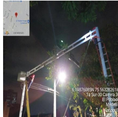
Ilustración 299 - LPR168, Instalación de cercha
