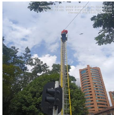
Ilustración 203 - P2140, Montaje de gabinete
