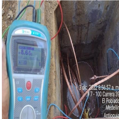
Ilustración 101 – P2155, Instalación puesta tierra
