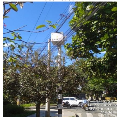
Ilustración 39 – LPR183, Instalación coraza, tierra y acometida
