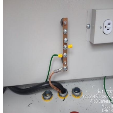
Ilustración 154 – LPR149, Conexión a tierra
