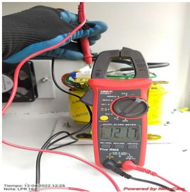
Ilustración 123 – LPR162, Instalación coraza
