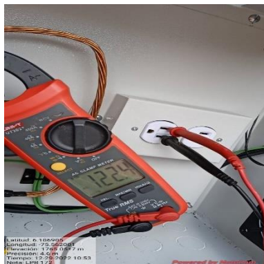
Ilustración 375 – LPR172, Energización de punto
