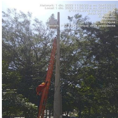
Ilustración 41 – P2157, Instalación brazo y coraza
