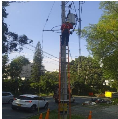
Ilustración 316 – LPR182, Búsqueda punto de conexión
