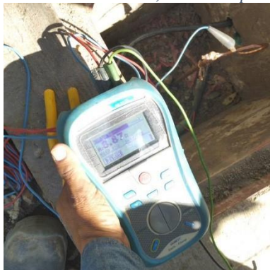
Ilustración 69 - LPR183, Puesta tierra
