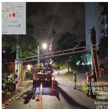
Ilustración 319 – LPR170, Instalación de cercha
