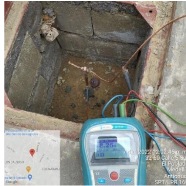
Ilustración 165 - LPR160, Instalación puesta tierra
