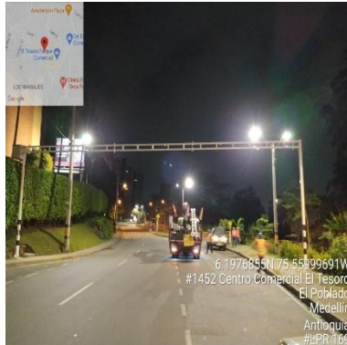
Ilustración 300 – LPR169, Instalación de cercha
