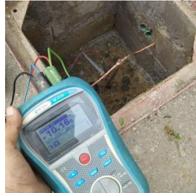
Ilustración 163 - LPR180, Instalación puesta tierra
