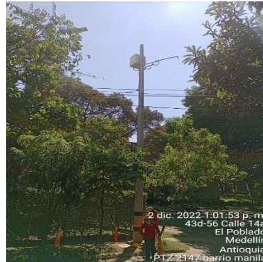
Ilustración 63 – P2147, Instalación brazo y coraza
