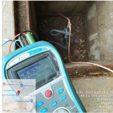
Ilustración 140 – LPR182, Instalación puesta tierra
