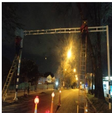
Ilustración 407 – LPR179, Cableado de cercha
