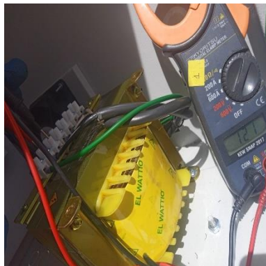
Ilustración 255 – LPR149, Energización de punto
