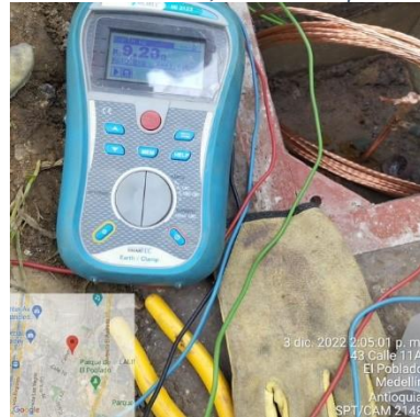
Ilustración 104 – P2148, Instalación puesta tierra
