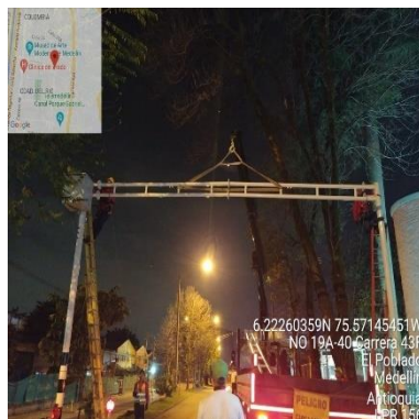
Ilustración 314 – LPR156, Instalación de cercha
