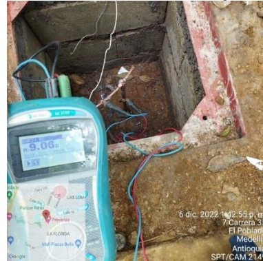
Ilustración 149 – P2149, Instalación puesta tierra
