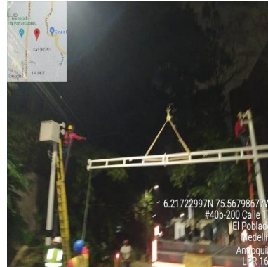
Ilustración 311 – LPR161, Instalación de cercha
