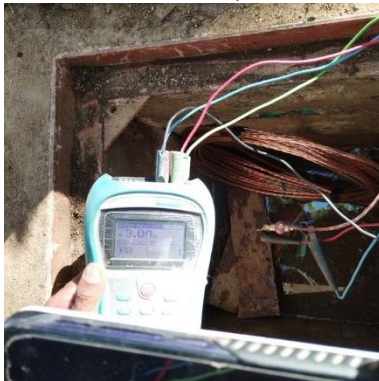
Ilustración 72 – P2157, Puesta tierra
