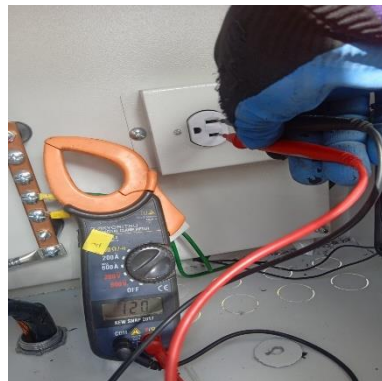
Ilustración 256 – LPR156 Energización de punto
