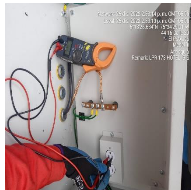
Ilustración 335 – LPR173, Energización de punto
