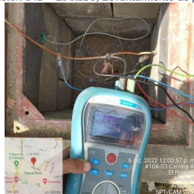
Ilustración 145 – P2153, Instalación puesta tierra
