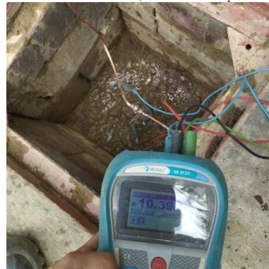
Ilustración 167 - LPR167, Instalación puesta tierra
