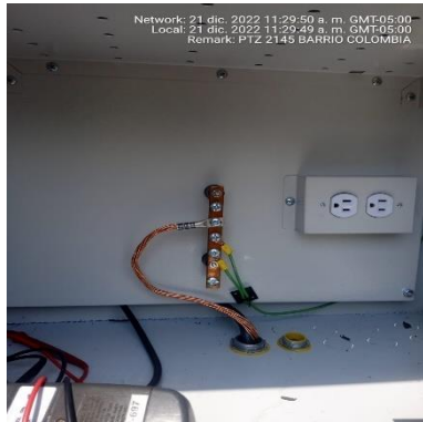
Ilustración 308 - P2145, Instalación de acometida
