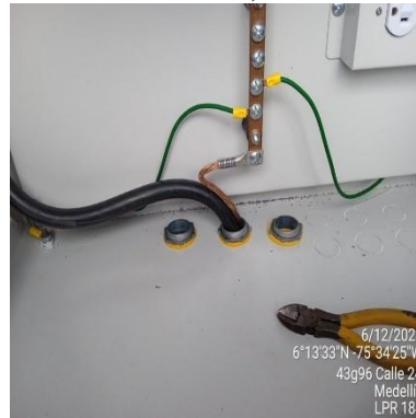
Ilustración 156 – LPR184, Conexión a tierra
