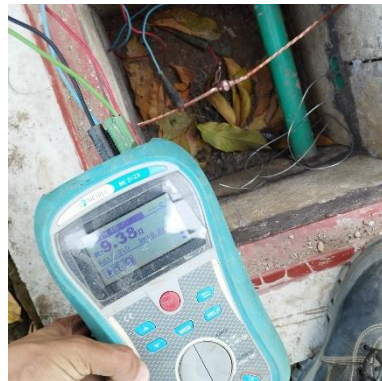
Ilustración 254 – LPR179, Instalación puesta a tierra
