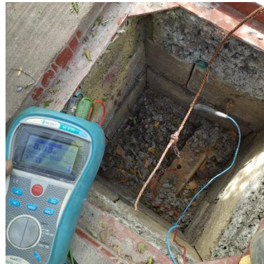
Ilustración 252 - P2164, Instalación puesta a tierra
