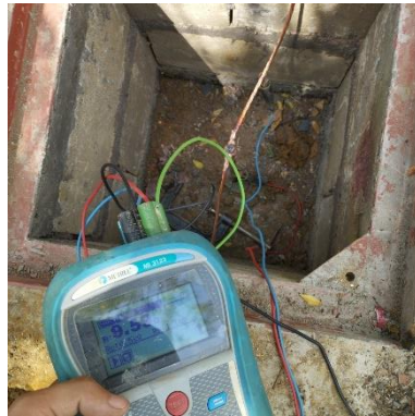
Ilustración 264 - LPR178, Instalación puesta a tierra
