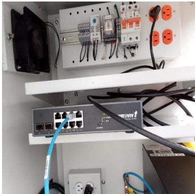
Ilustración 23 – LPR173, Instalación de switch
