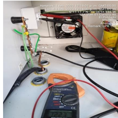
Ilustración 10 – LPR163, Energización de punto
