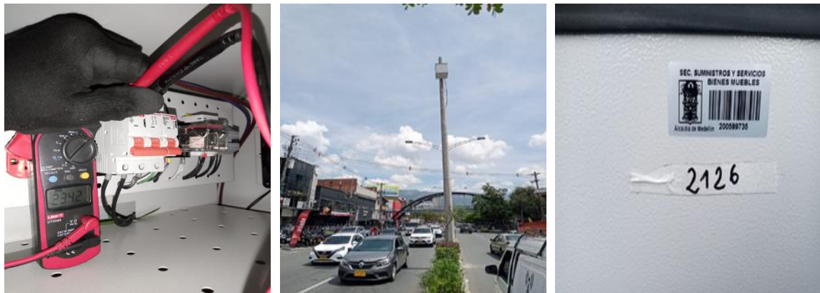
Ilustración 213 Instalación de gabinete y energización de punto 2126.
