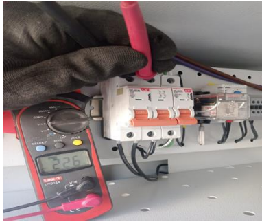
Ilustración 184 Instalación de gabinete y energización de punto 2077.
