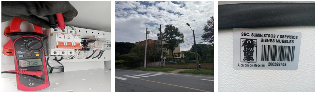
Ilustración 214 Instalación de gabinete y energización de punto 2127.
