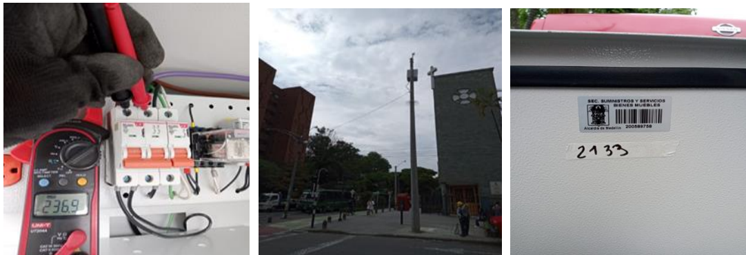
Ilustración 217 Instalación de gabinete y energización de punto 2133.
