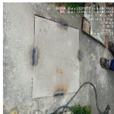
Ilustración 172 - P2165, Soldadura de caja
