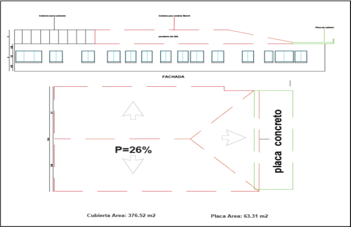
CORTE FACHADA
