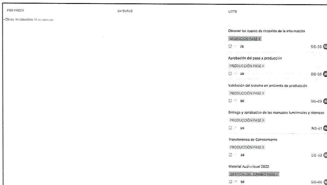
Ilustración. 7 Sprint activo 1
