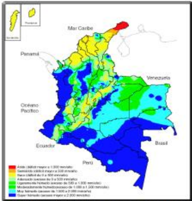
Figura 6. Zonificación de suelos por humedad: árido (rojo), semiárido (ocre), seco (amarillo), adecuado (amarillo verdoso), ligeramente húmedo (verde claro), moderadamente húmedo (verde), muy húmedo (azul claro), súper húmedo (azul oscuro). Fuente: www.todacolombia.com
