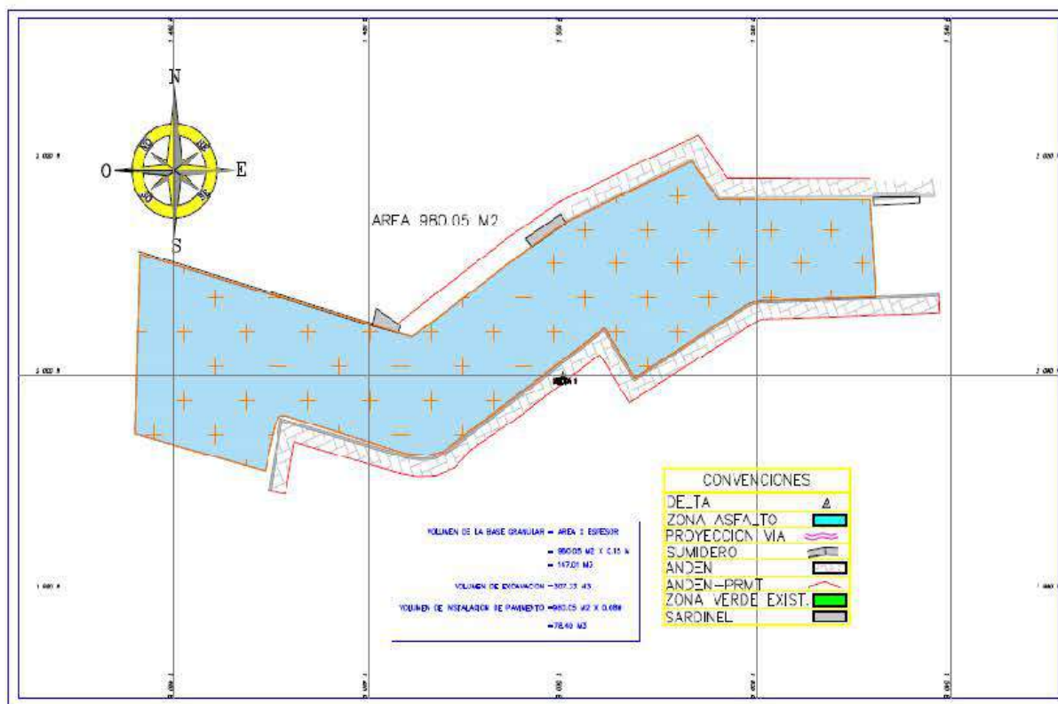
Figura 2. Levantamiento topográfico Sector La Gran Ladera con las áreas de volúmenes de excavación, base granular y asfalto.
