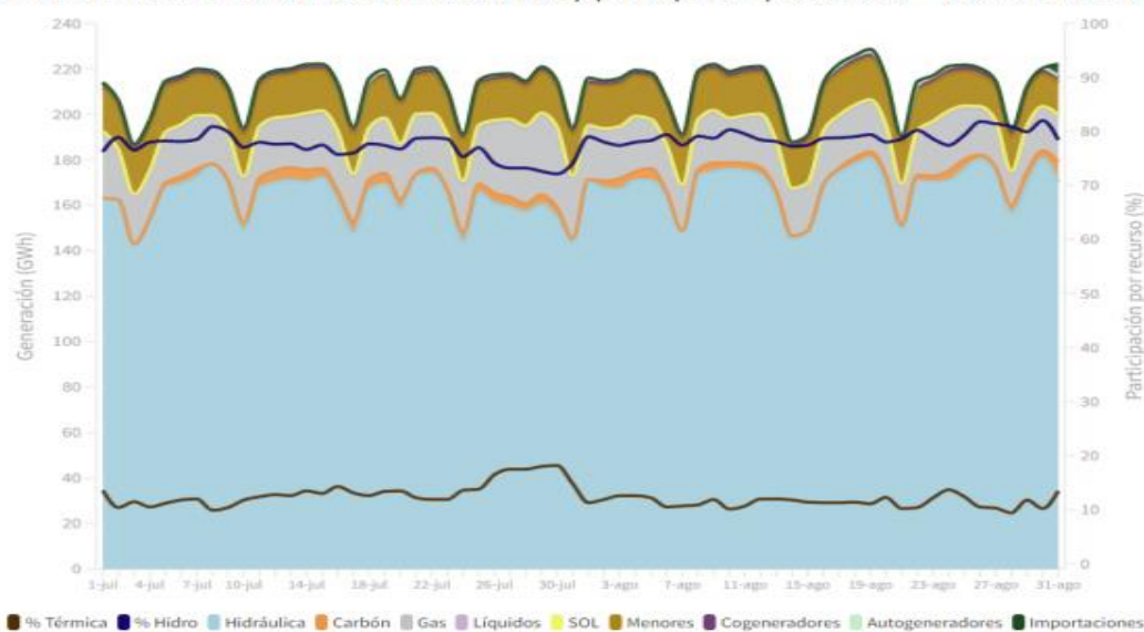
Ilustración 3. Generación de electricidad del SIN y participación por recurso – último bimestre (GWh)
