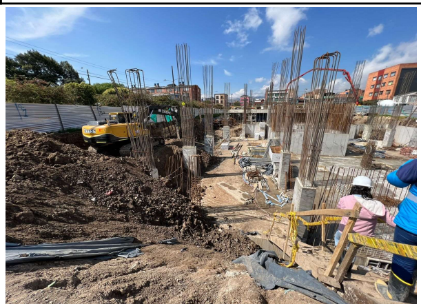
BLOQUE B - SOTANO
