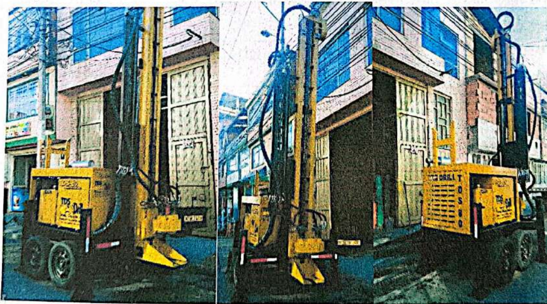
Imagen 1. Equipo de perforación TDS 100 POWER HYDRAULICS
